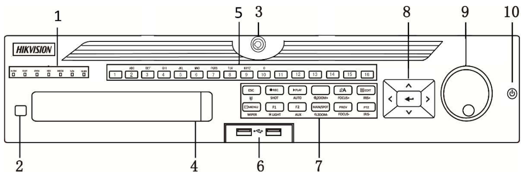
Rysunek 1-4: Panel przedni modelu DS-9000HUHI-K8 i iDS-9016HUHI-K8/16S
