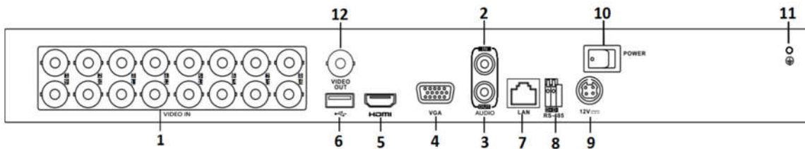
Rysunek 1-12: Panel tylny DS-7200HQHI-K (z 16 wejściami wideo)
