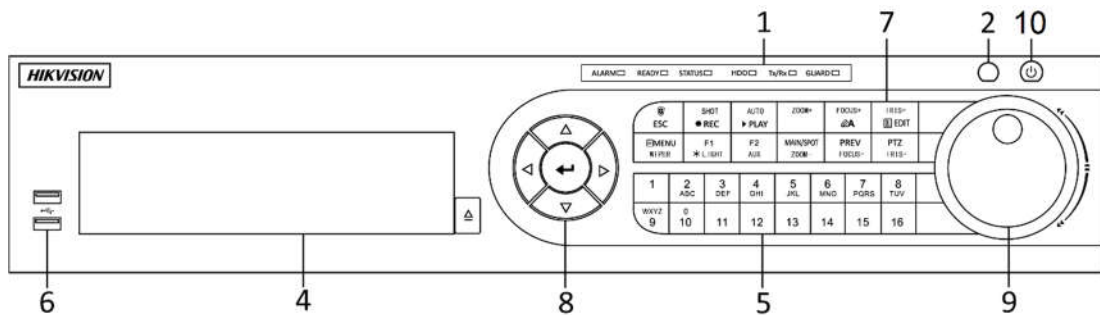
Rysunek 1-3: Panel przedni DS-8100HQHI/HUHI-K8
