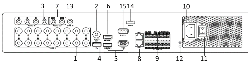
Rysunek 1-16: Panel tylny DS-7300HUHI-K4 (z 16 wejściami wideo)
