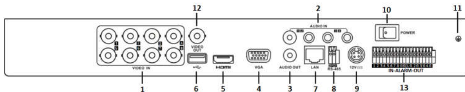
Rysunek 1-11: Panel tylny DS-7200HTHI-K2
