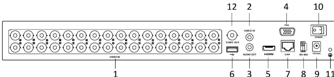
Rysunek 1-13: Panel tylny DS-7200HQHI-K (z 32 wejściami wideo)
