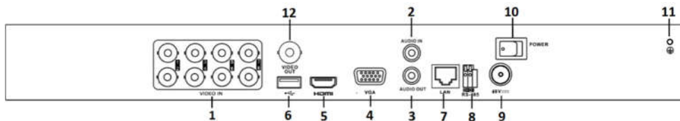
Rysunek 1-14: Panel tylny DS-7200HQHI-K/P
