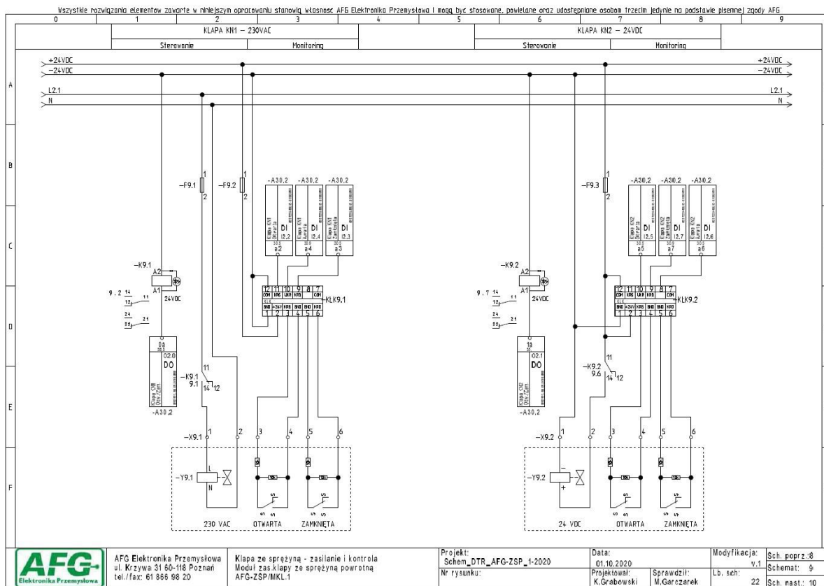
Rysunek 3.9. SCHEMAT MODUŁU ZASILANIA i KONTROLI KLAPY ze SPRĘŻYNĄ POWROTĄ – AFG-ZSP/MKL.1
